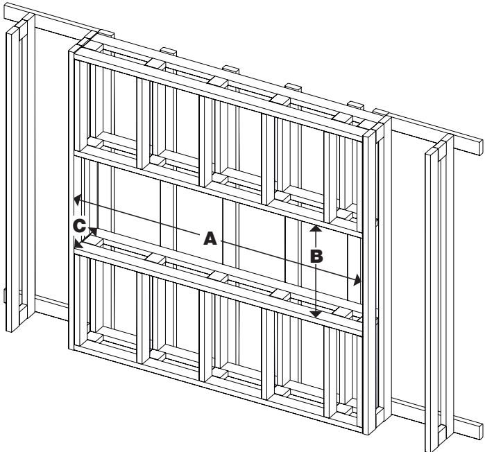
Figura 10 Instalación frontal
