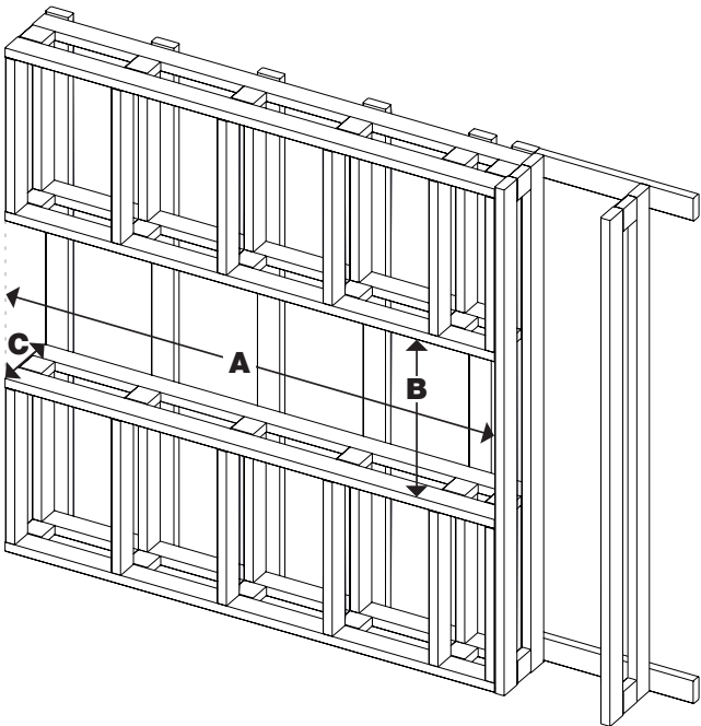
Figura 9 Instalación en esquina izquierda o derecha
